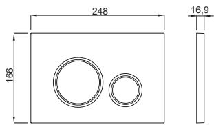
Schiță tehnică
