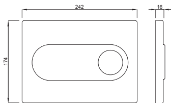
Schiță tehnică
