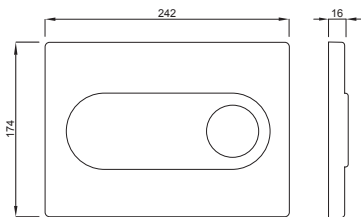
Schiță tehnică
