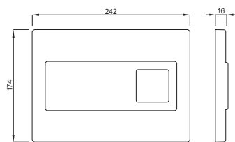
Schită tehnică
