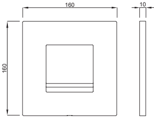
Schița tehnică
